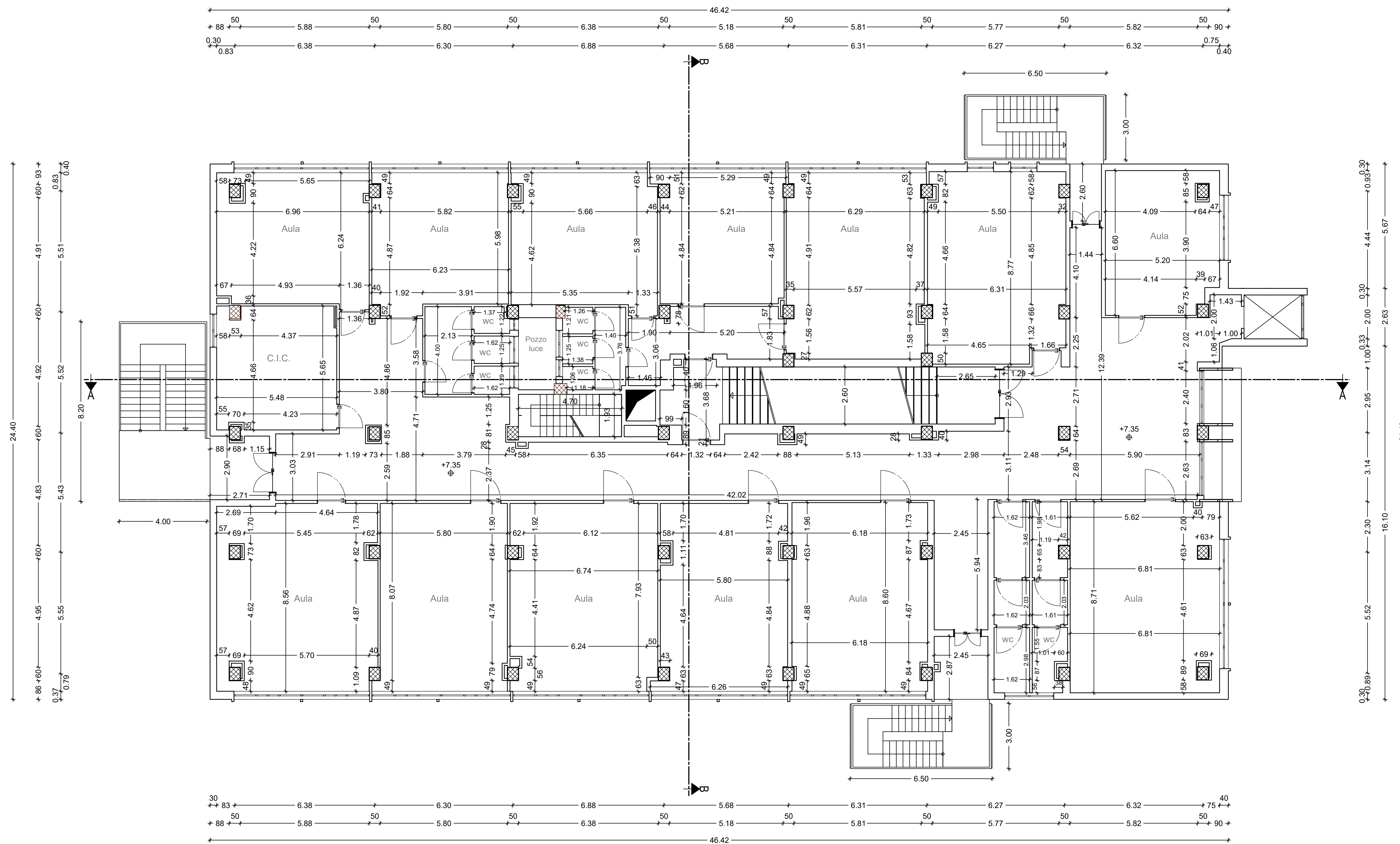
PIANTA PIANO SECONDO
