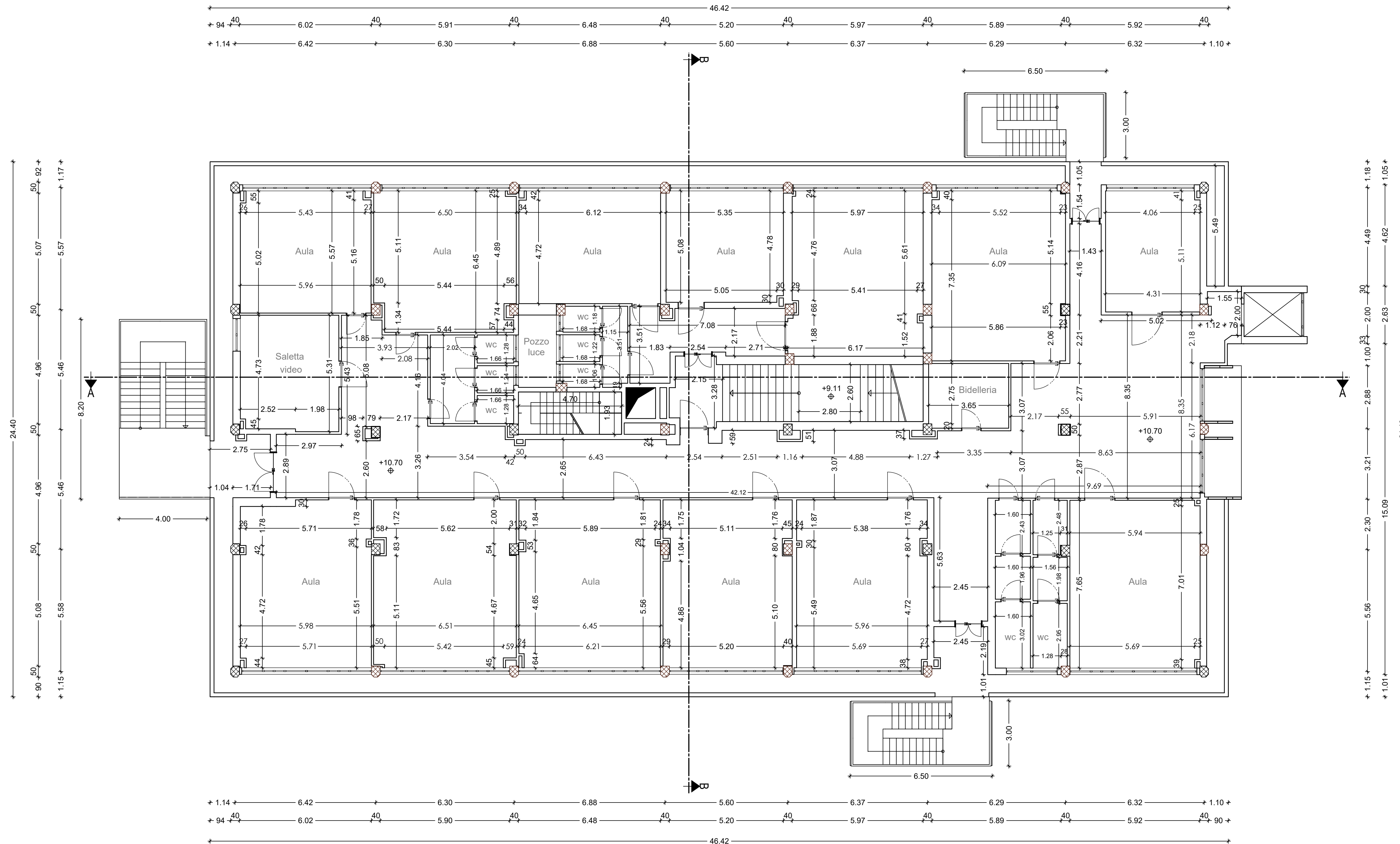
PIANTA PIANO TERZO
